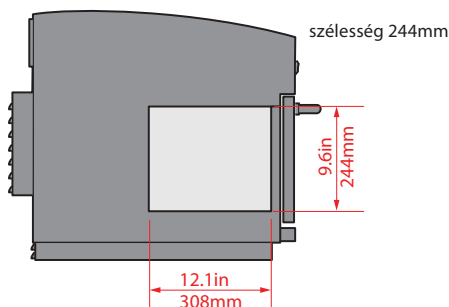
Sütőkamra méretei
