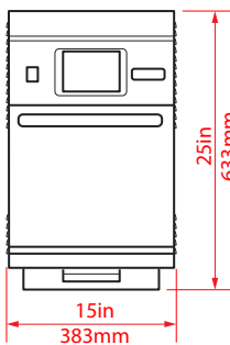
Sütő méretei
